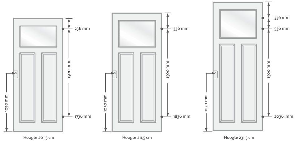
Positie slotgat en paumelleboringen.
