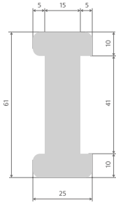
AANSLAGLAT FACET PROFIEL T.B.V. DUBBELE SCHUIF- DEUREN
