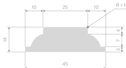
Aanslaglat Kraal profiel
