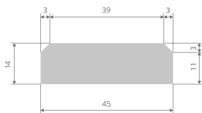
AANSLAGLAT FACET PROFIEL
