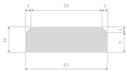
Aanslaglat Facet profiel
