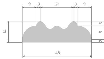
AANSLAGLAT DUBBEL KRAAL PROFIEL
