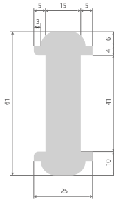
AANSLAGLAT KRAAL PROFIEL T.B.V. DUBBELE SCHUIFDEUREN
