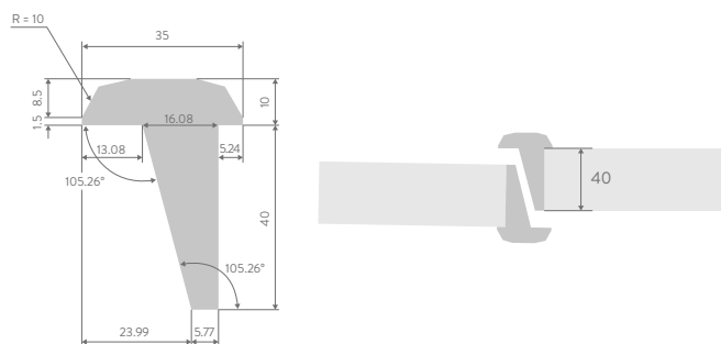
TONGNAALD T.B.V. DUBBELE STOMPE DEUREN
