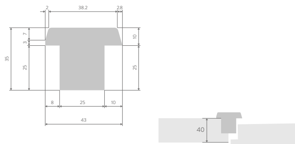
Tongnaald t.b.v. dubbele opdekdeuren
