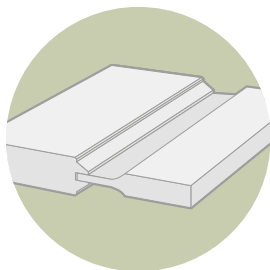
facet profiel - traditioneel paneel
