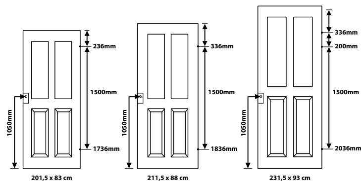
Positie paumelle gaten (standaardhoogtes)
