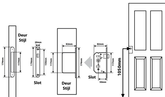
Positie slotgat (standaard)
